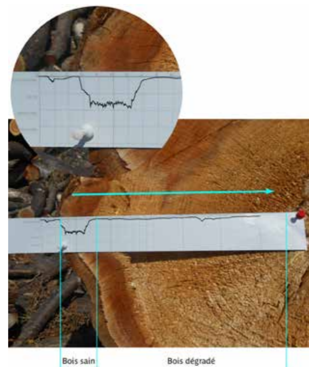
Courbe de résistance du bois :
